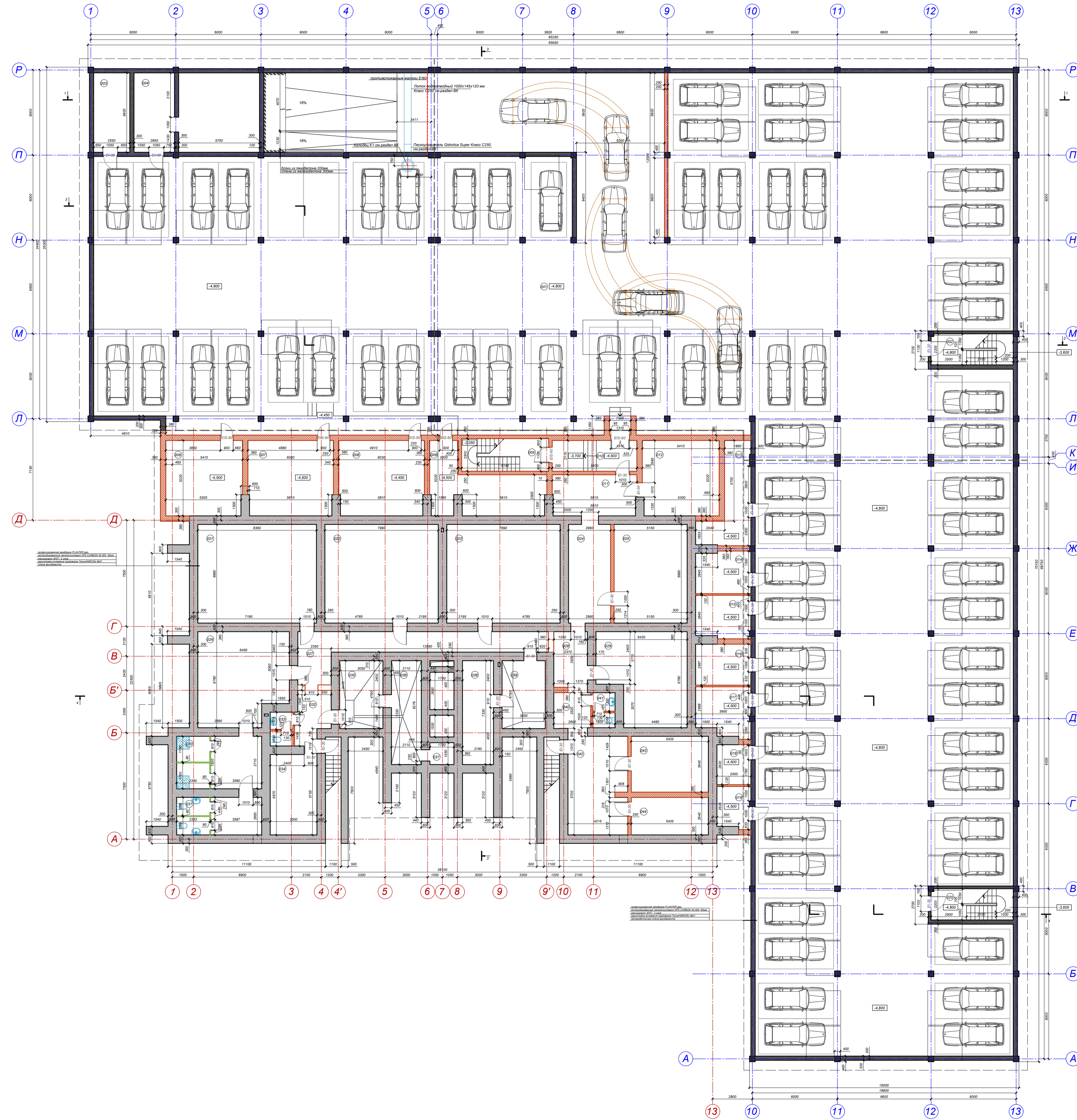
План на отметках -4.900, -4.500, -2.770. М1:75
