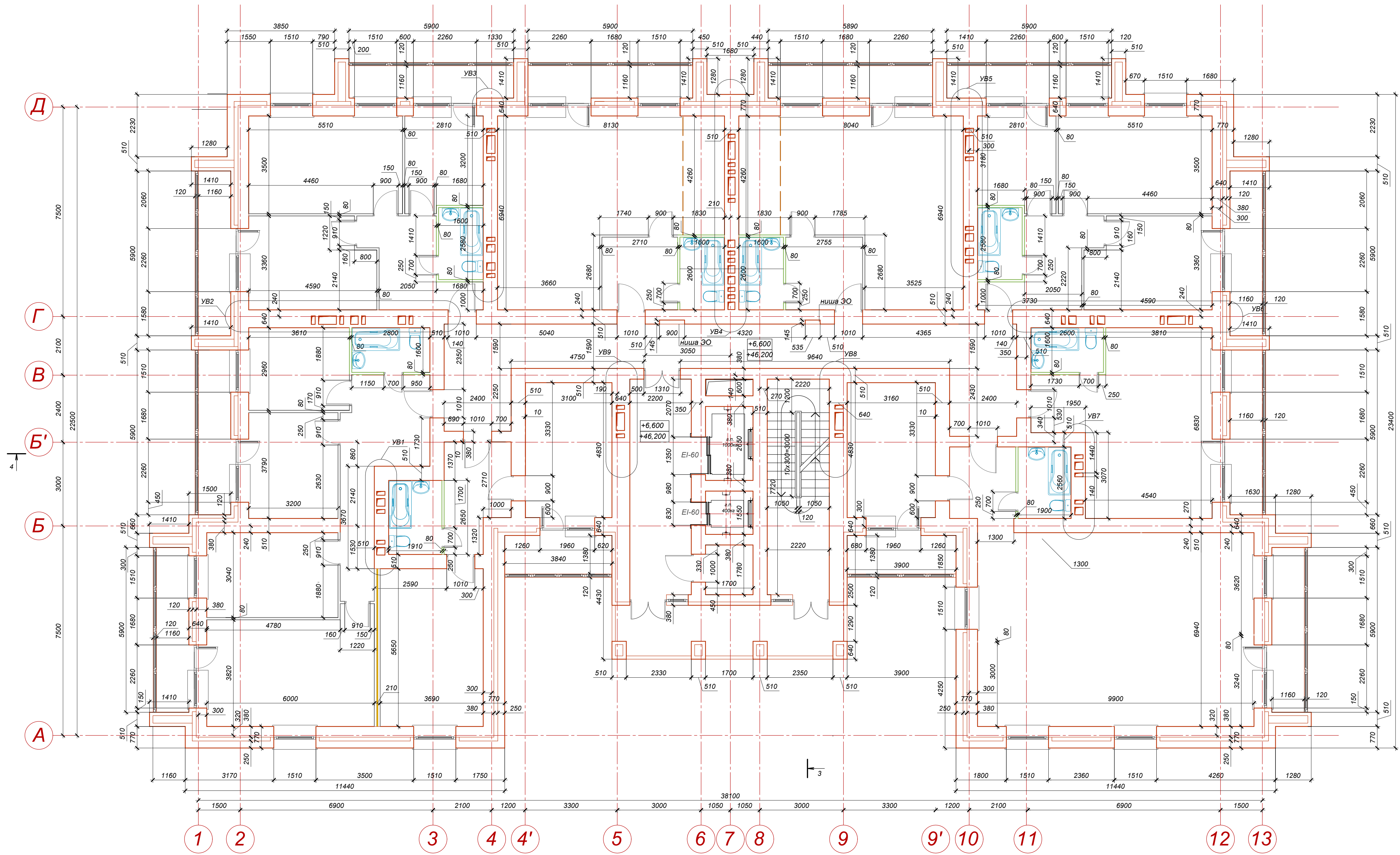
План на отметках +6,600 -- +46,200 ( типовые этажи ). М1:75
