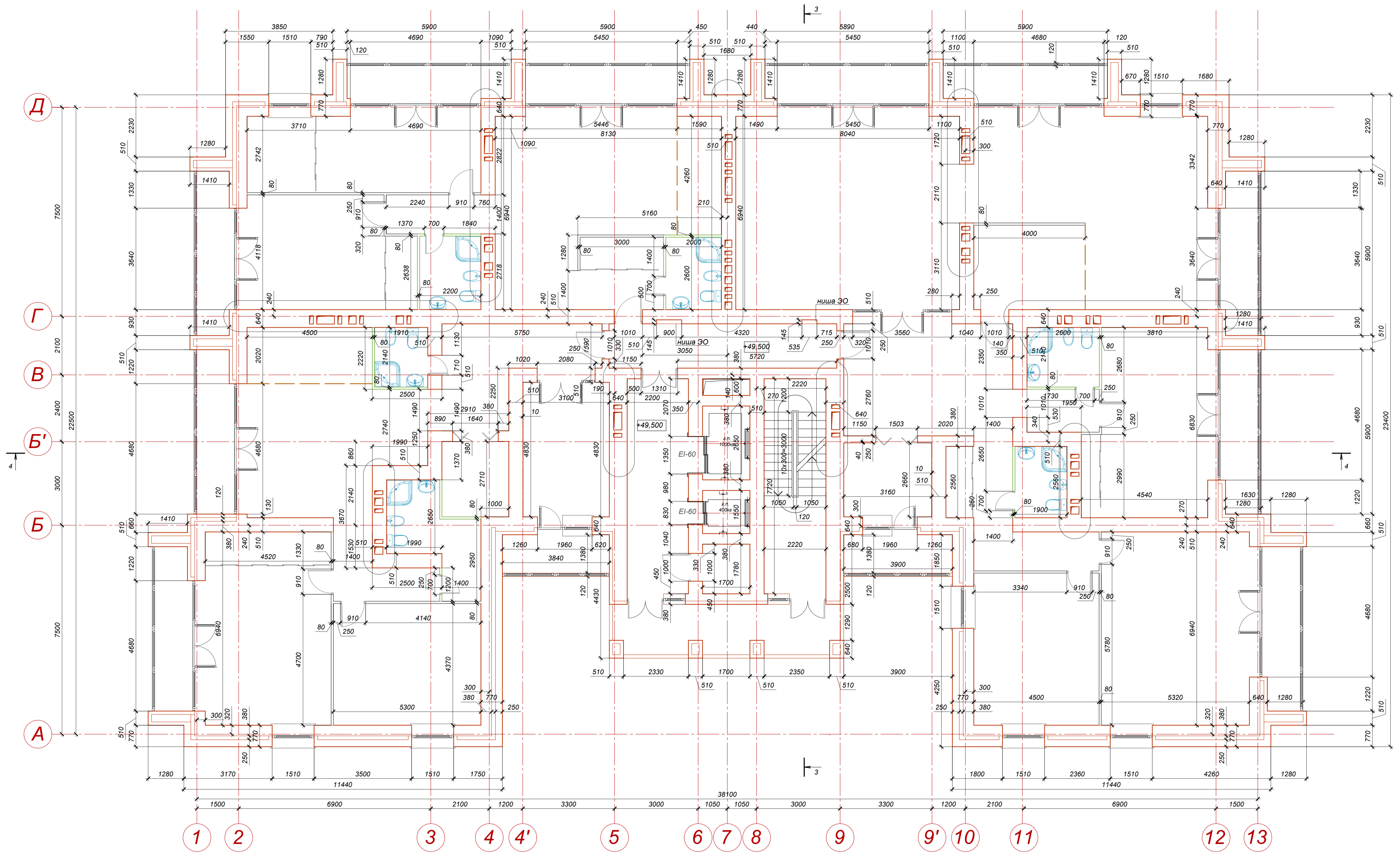
План на отметках +49,500 (16 этаж). М1:75
