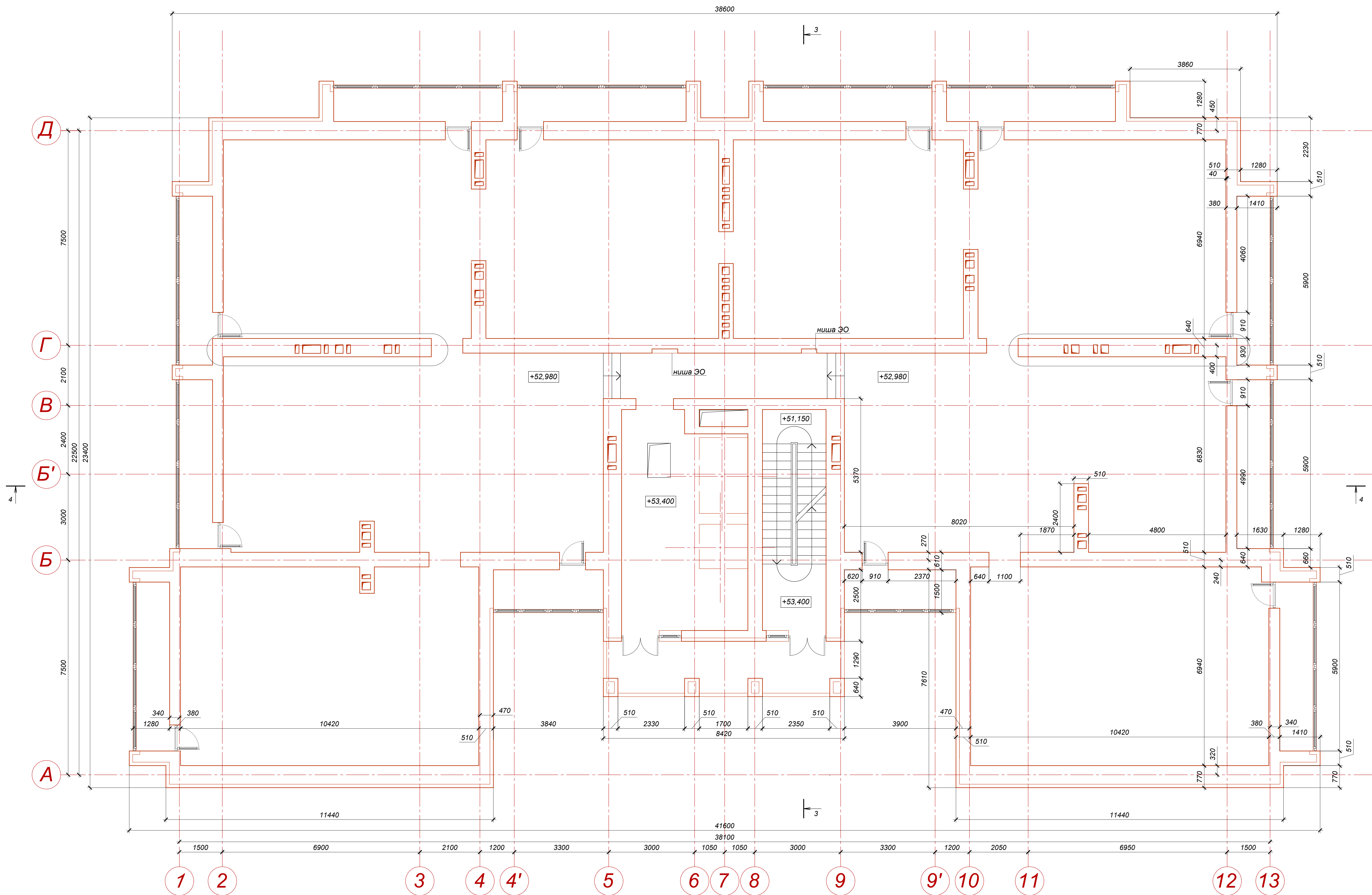
План на отметках +52,980 (17, технический этаж). М1:75
