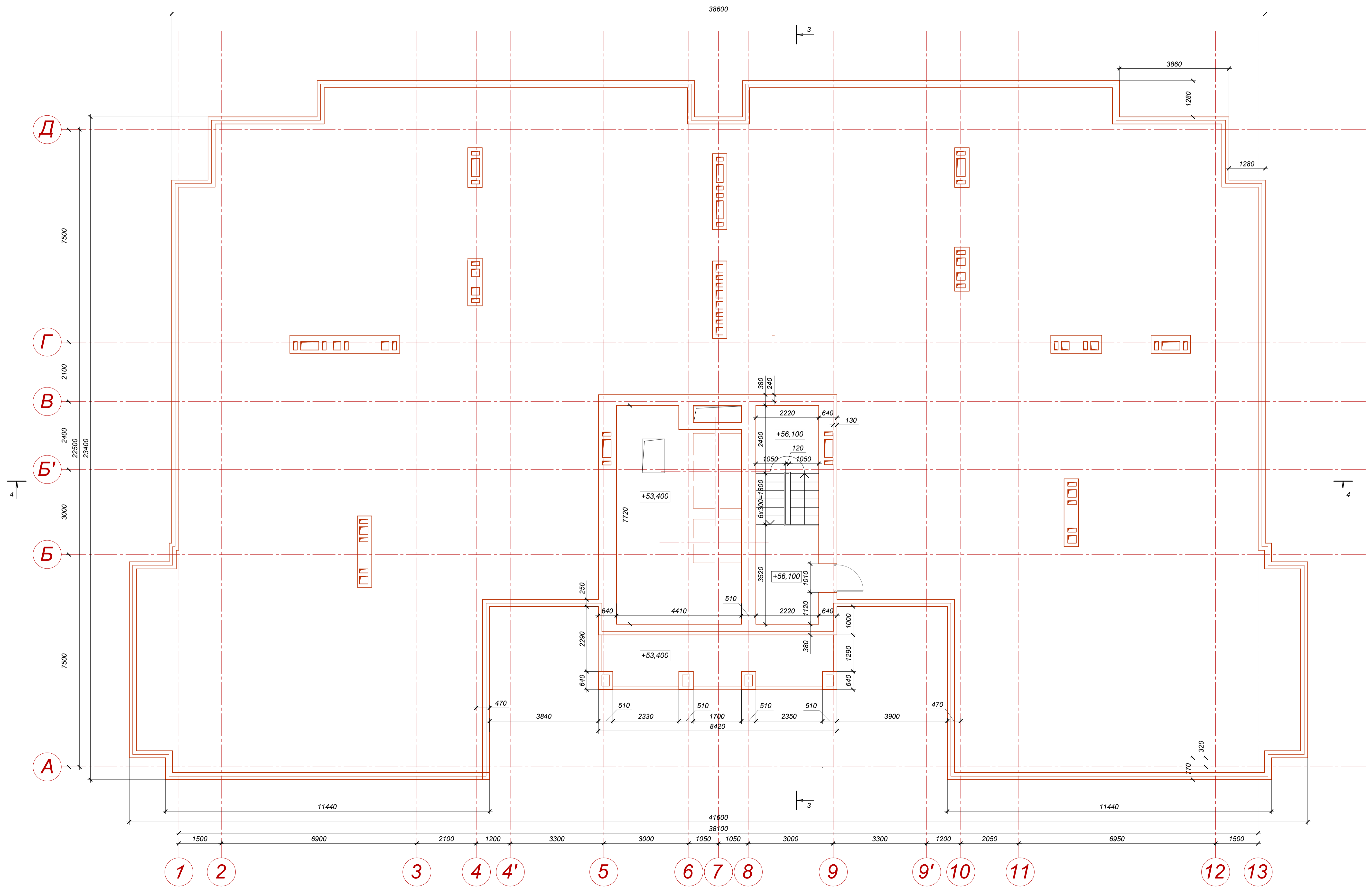
План на отметках +55,920 (кровля). М1:75
